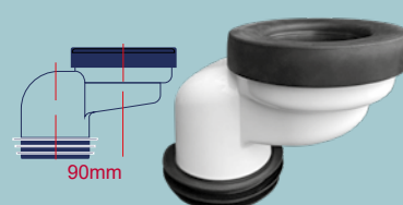
NUEVO Manguito WC Excéntrico 90mm Cod. 61068 Excéntrico (hasta 90mm)
