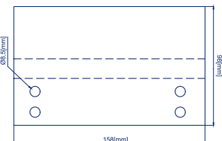
Uñeta Larga para Fijación de Lavamanos
