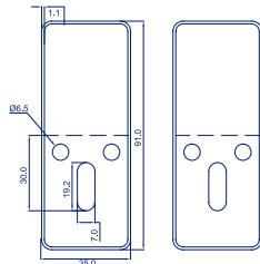
Uñeta Doble Fijación para Lavamanos
